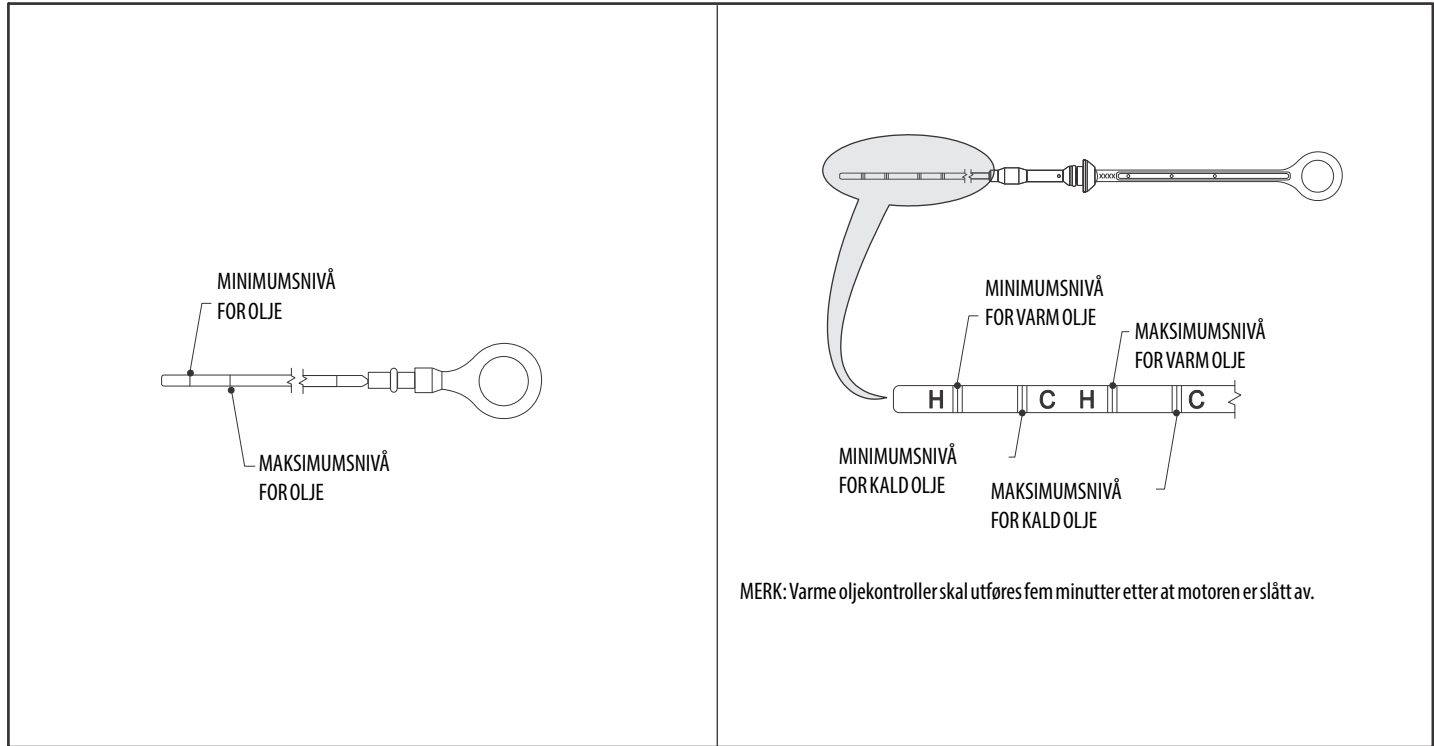
Figur 7-7. Deutz 2011-motorpeilepinne
