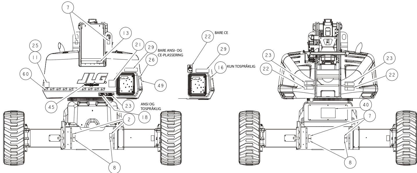
Figur 4-12. Merkeplassering – ark 5 av 7
