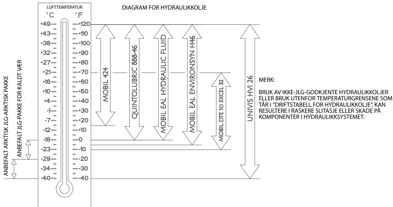
Figur 7-2. Diagram for hydraulikkolje – ark 1 av 2
