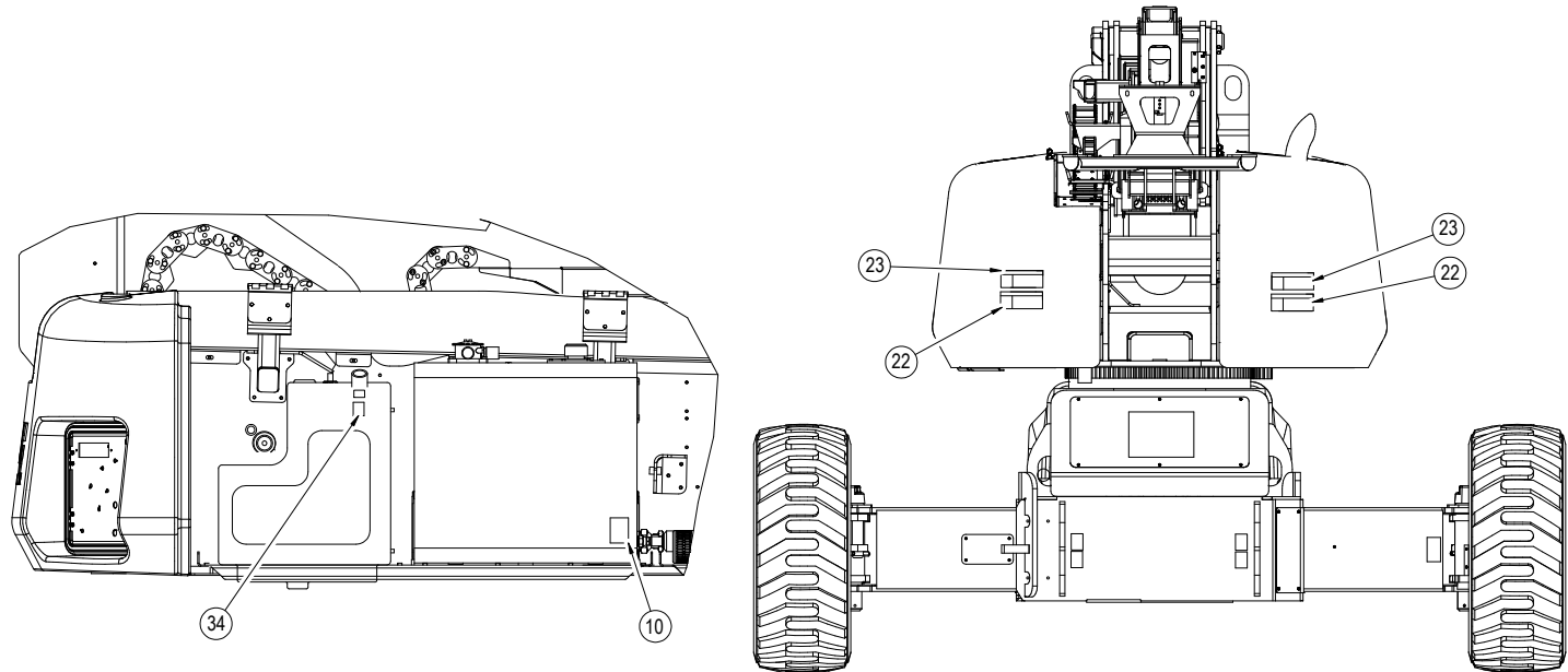
Figur 4-14. Merkeplassering – ark 7 av 7
