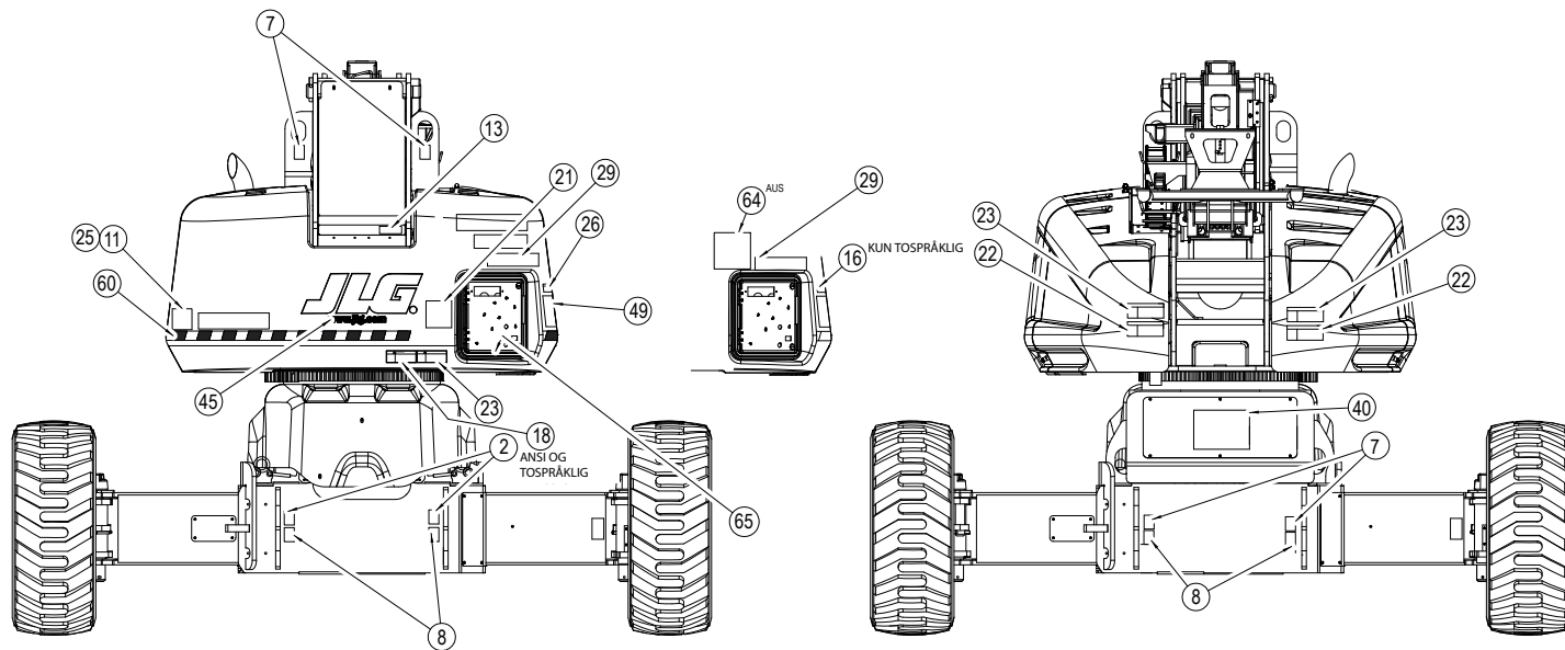
Figur 4-19. Merkeplassering (Bare CE) – SN 0300141473 til nåværende – Ark 5 av 6
