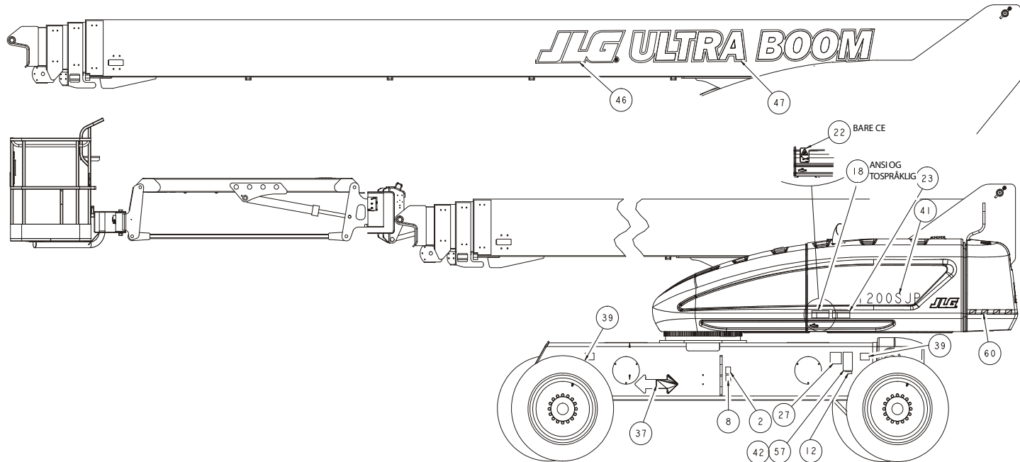
Figur 4-8. Merkeplassing – ark 1 av 7
