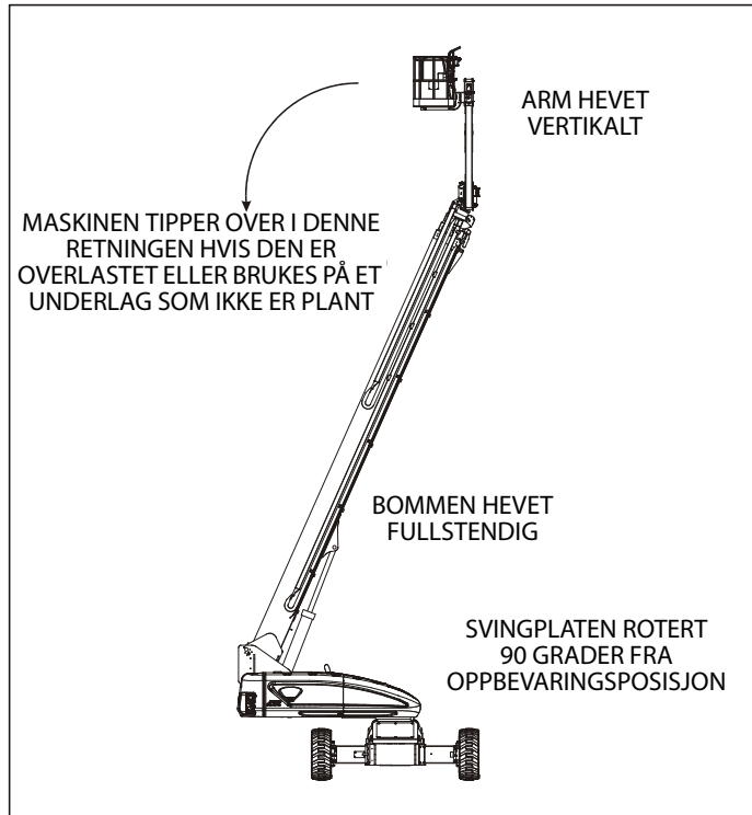
Figur 4-3. Posisjon med minst stabilitet bakover
