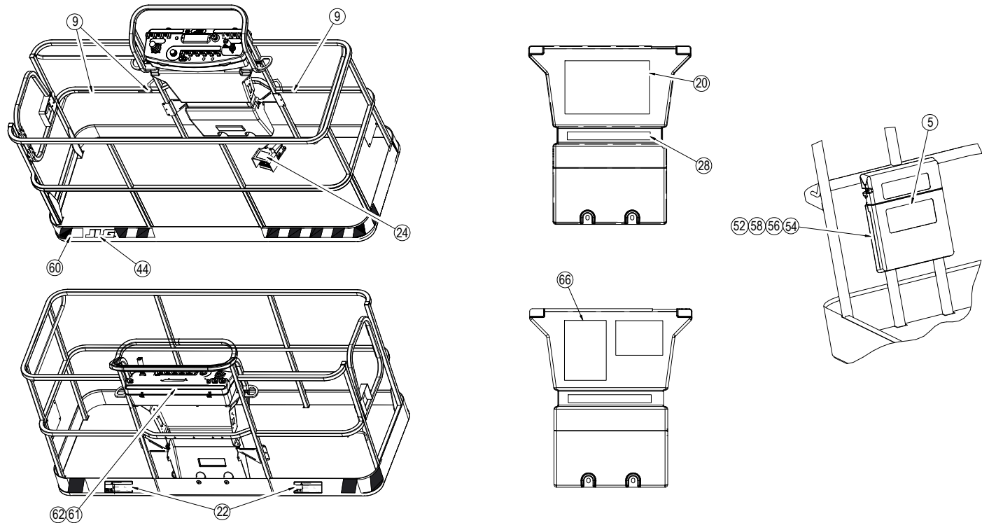
Figur 4-16. Merkeplassering (Bare CE) – SN 0300141473 til nåværende – Ark 2 av 6
