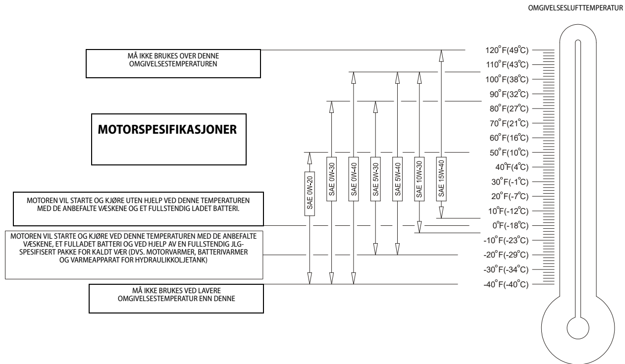
Figur 7-4. Spesifikasjoner for motorens driftstemperatur – Caterpillar – ark 1 av 2
