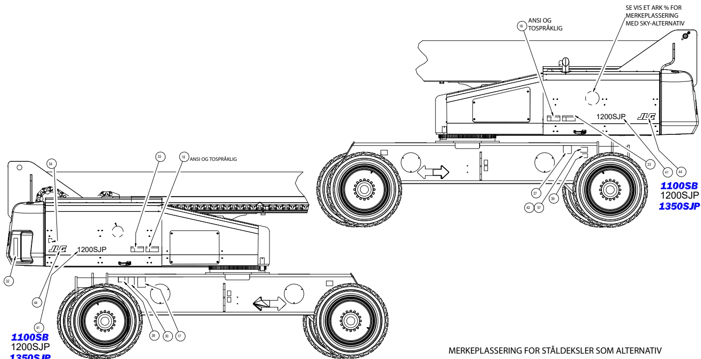
Figur 4-13. Merkeplassingering – ark 6 av 7
