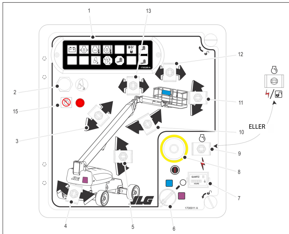
Figur 3-1. Bakkekontrollstasjon
