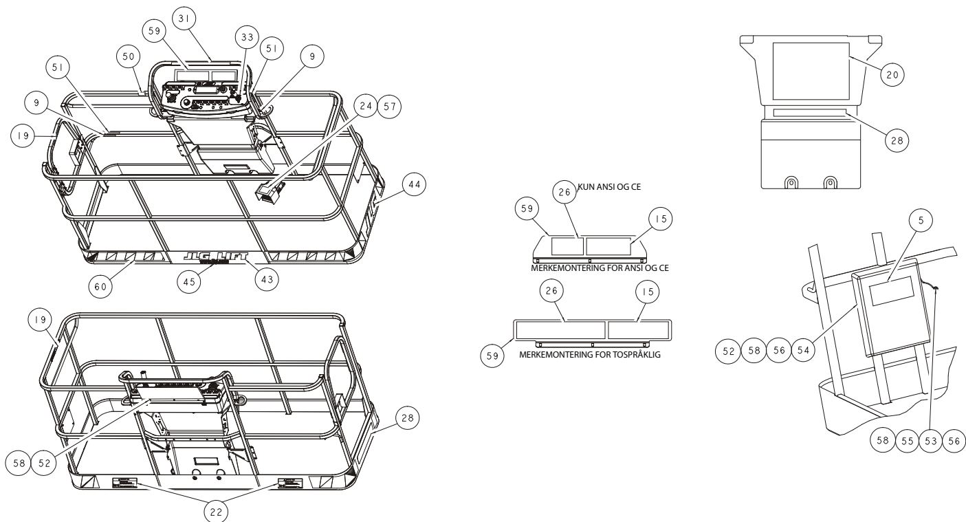
Figur 4-9. Merkeplassering – ark 2 av 7
