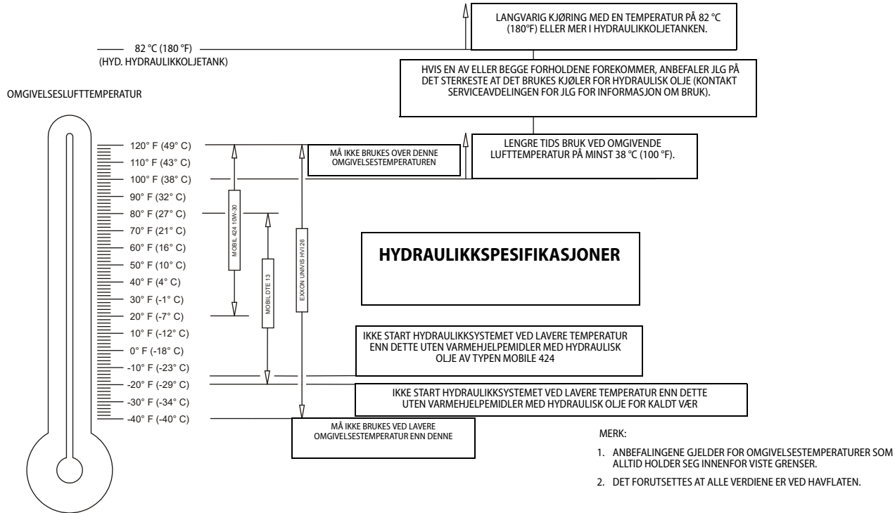
Figur 7-5. Spesifikasjoner for motorens driftstemperatur – Caterpillar – ark 2 av 2
