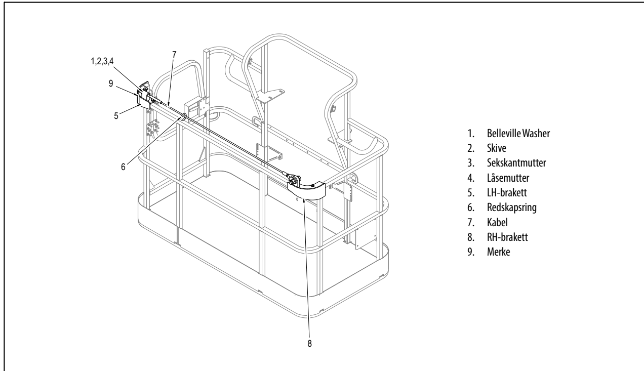
Figur 6-2. Eksternt "bolt-på"-fallsikringssystem
