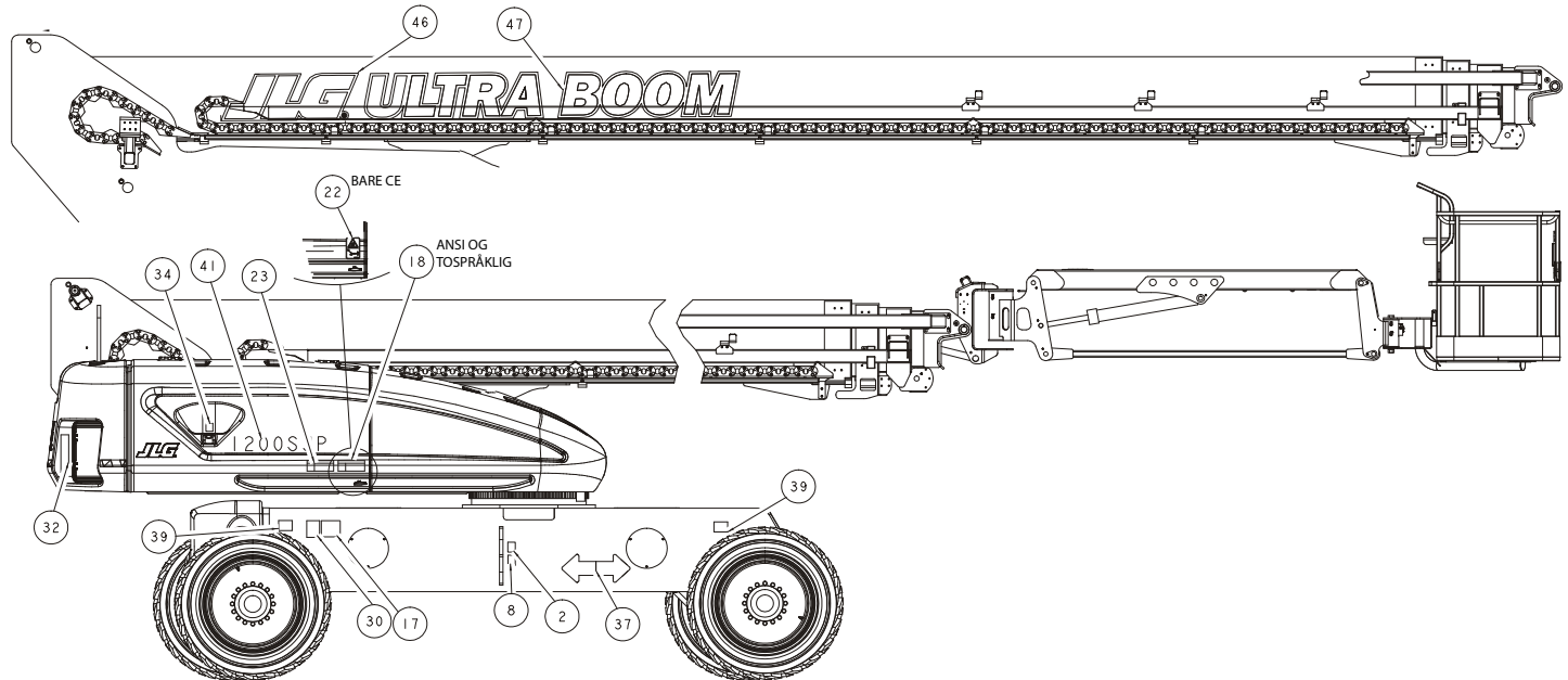
Figur 4-10. Merkeplassing – ark 3 av 7
