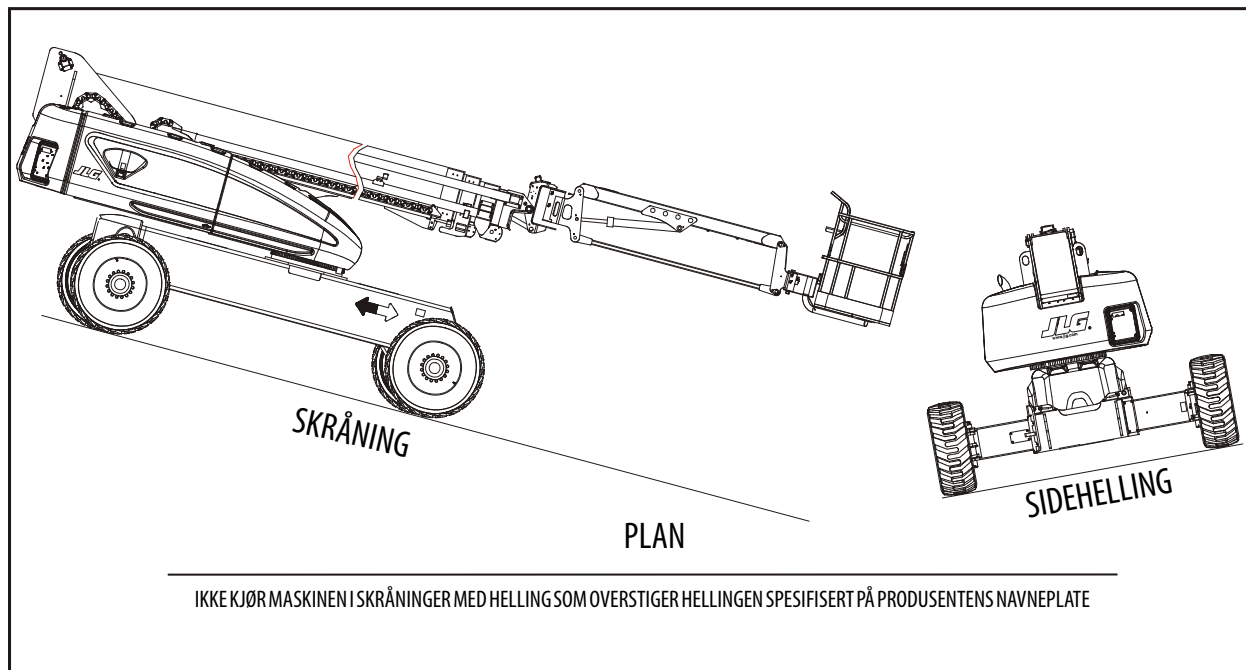
Figur 4-5. Skråning og sidehellinger
