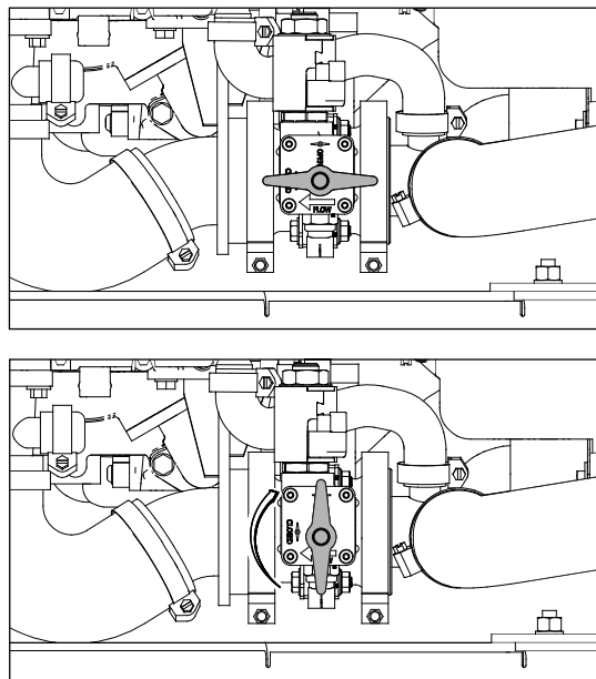
Figur 4-1. ASOV-tilbakestilling (åpen til lukket posisjon)
