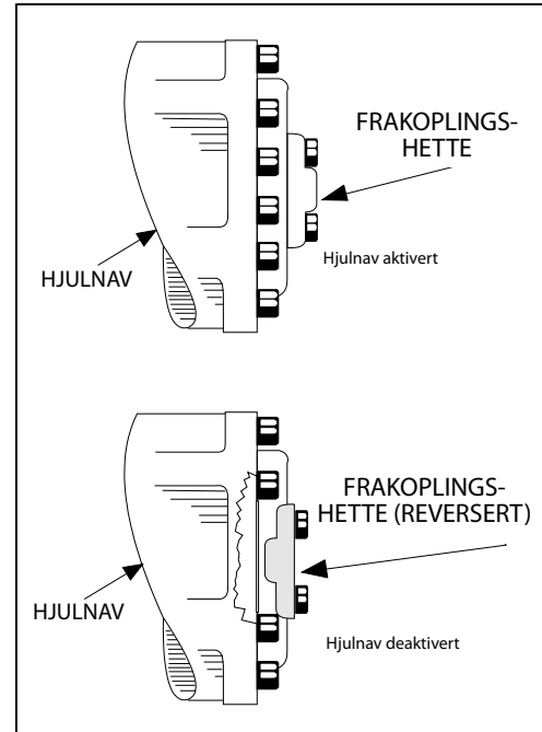
Figur 4-6. Kjøreutkoplingsnav
