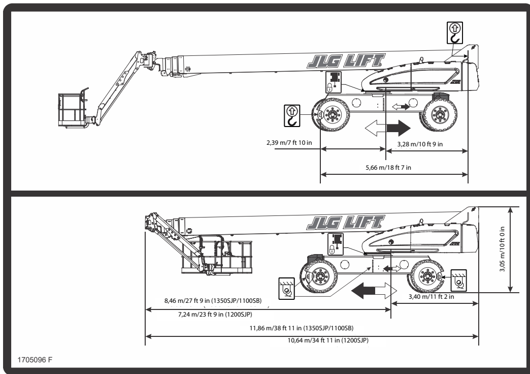
Figur 4-7. Løfte- og festediagram
