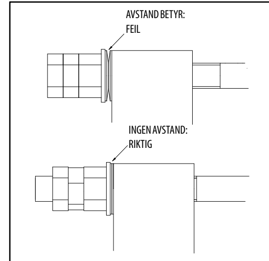
Figur 6-1. Stramming av kabel i det eksterne "bolt-på"-
