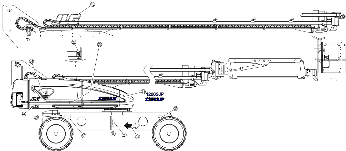
Figur 4-17. Merkeplassering (Bare CE) – SN 0300141473 til nåværende – Ark 3 av 6
